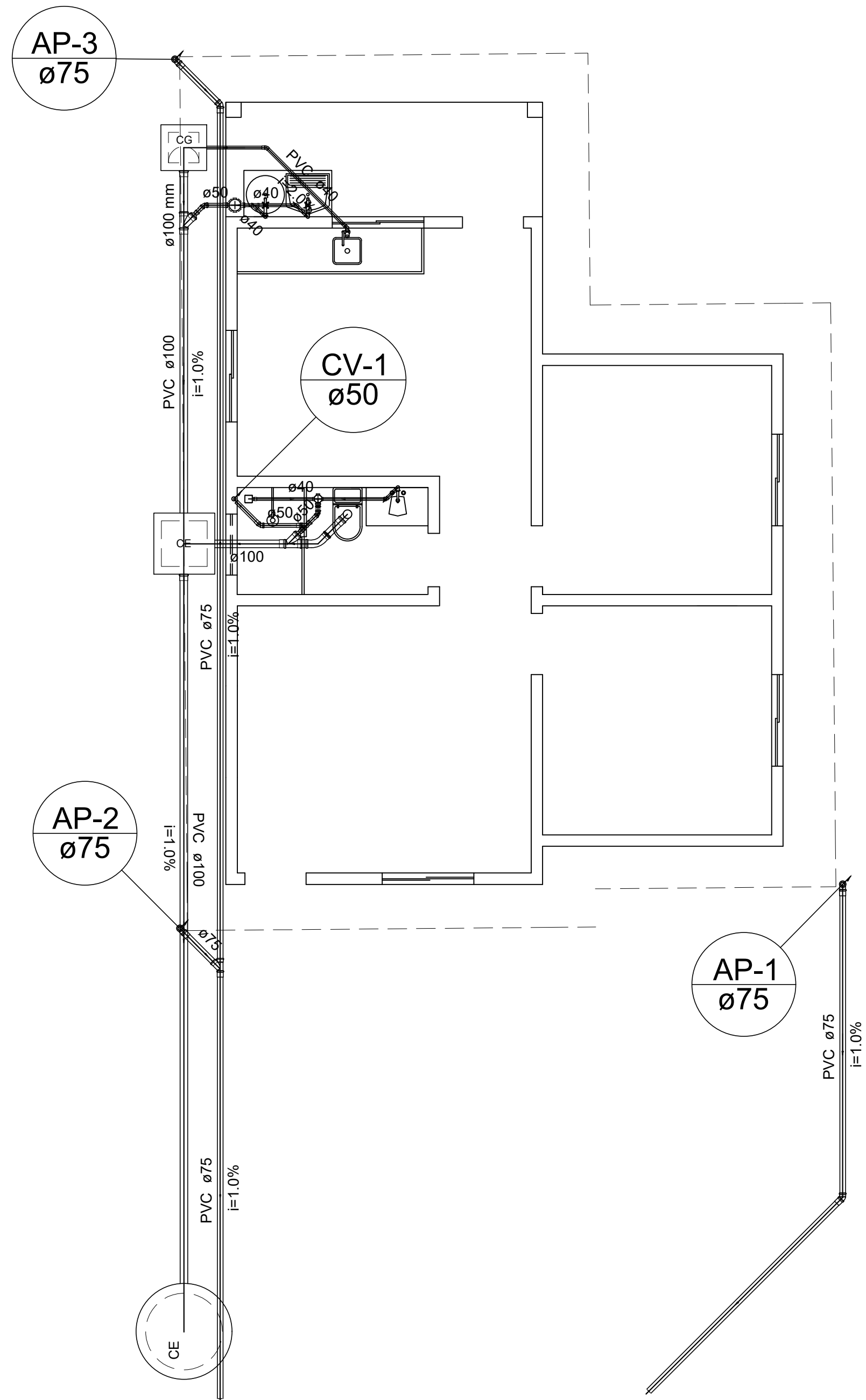
Detalhe S1 escala 1:50
