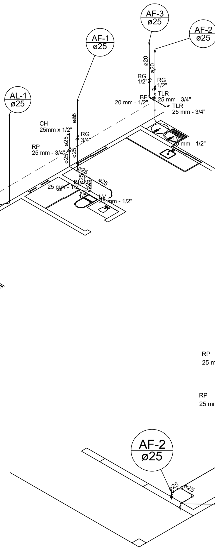
Detalhe H2 escala 1:50
